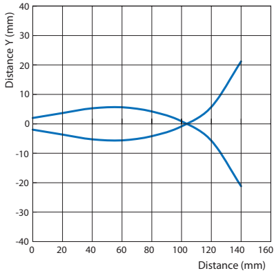
E3FN-P 18KDR 1
