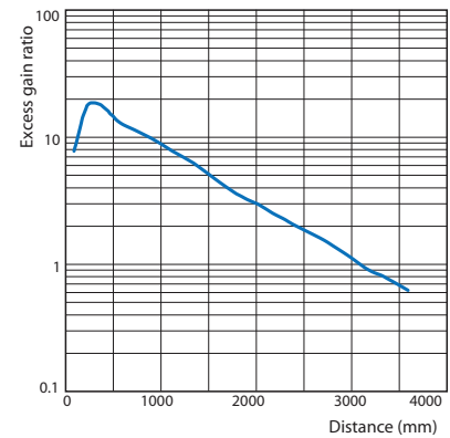
E2FN-P 18KR 2
